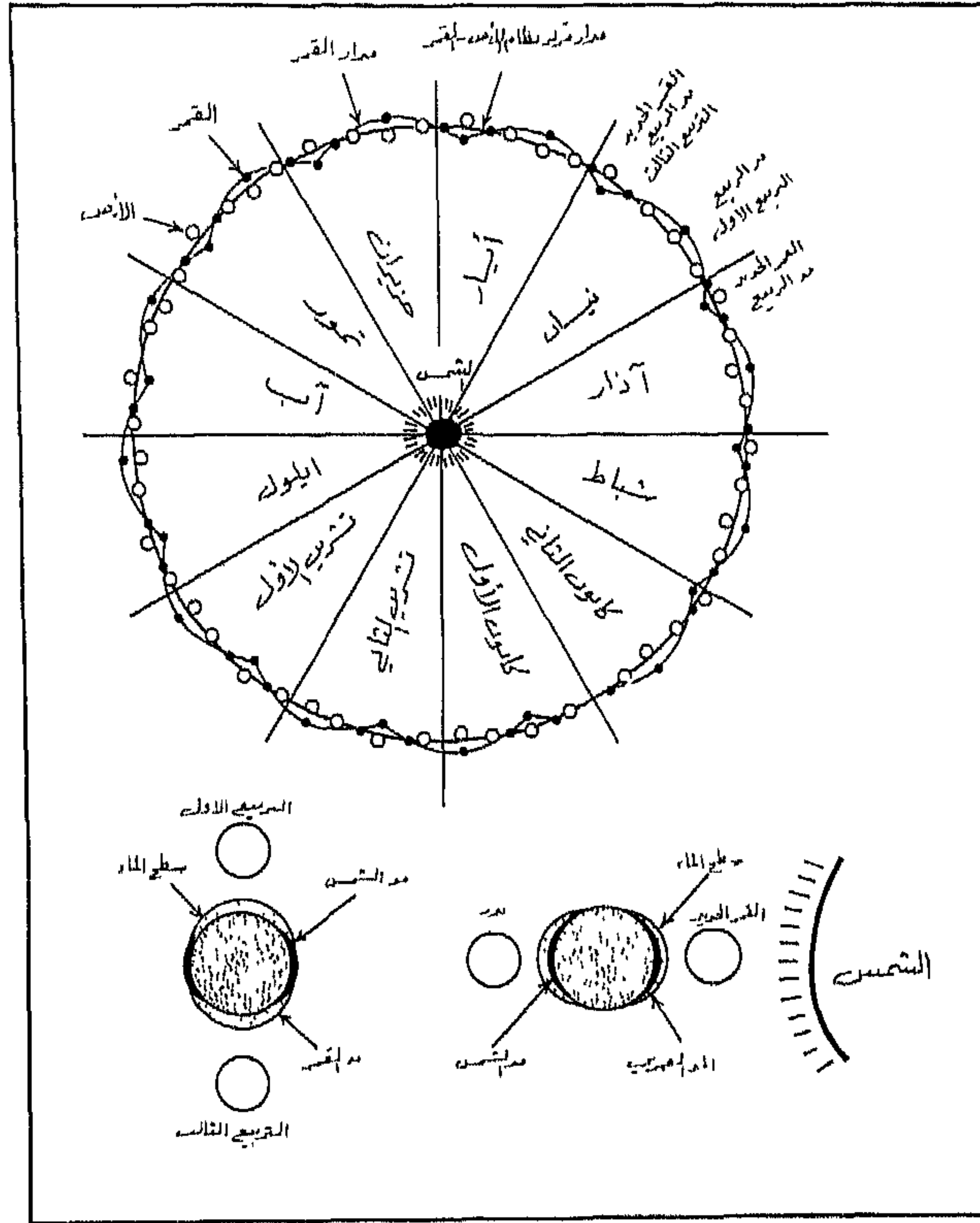
شكل (57) العلاقة بين المد ومنازل القمر
